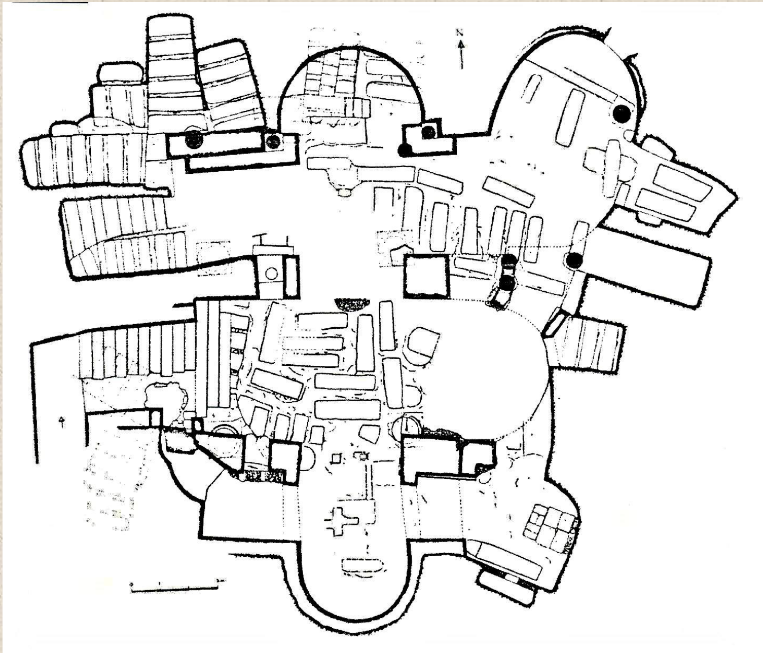
Cripta di S. Marciano, planimetria
