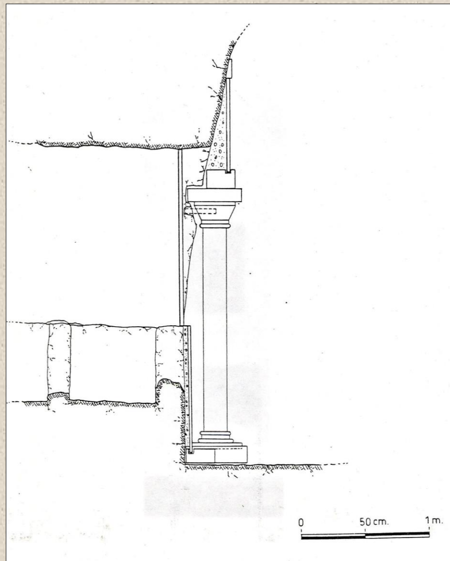
Rotonda di Adelfia, arcosolio anonimo: 1. prospetto; 2. sezione
