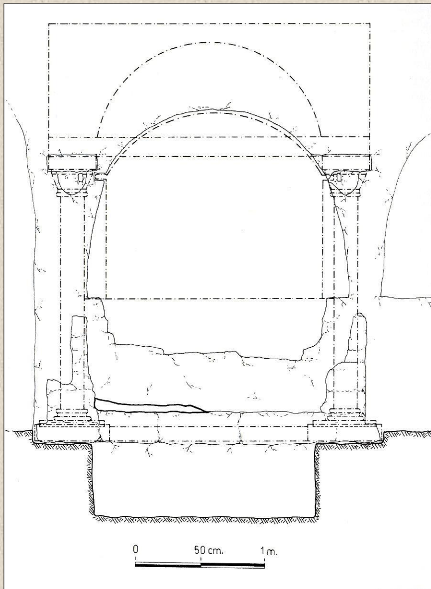
Rotonda di Adelfia, arcosolio anonimo: 1. prospetto; 2. sezione
