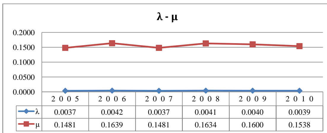
Слика 44 - Интензитети отказа и поправки
