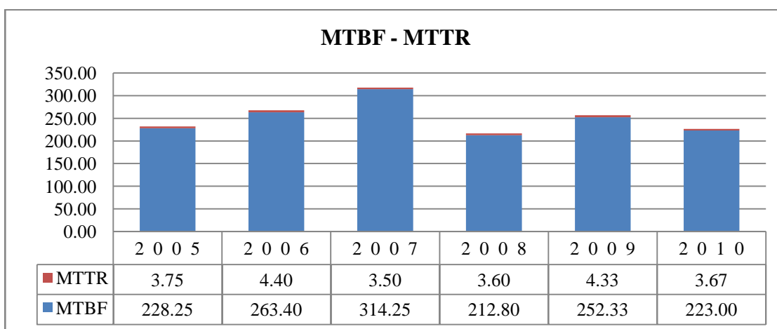
Слика 73 - Однос средњих времена отказа и поправки
