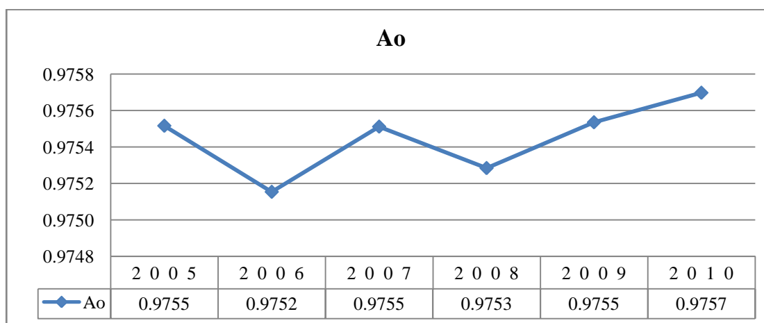
Слика 39 - Функција расположивости
