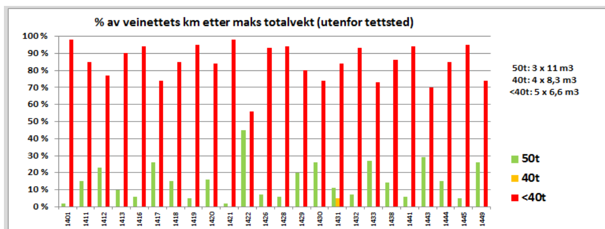
Figur 2. Andelen av det kommunale veinettet klassifisert etter tillatt totalvekt (50 t, 40 t, < 40 t) med angitt kippealternativ for bil uten henger (totalvekt: antall turer og nyttelast). Etter Molstad (2018).
