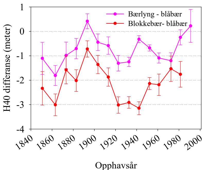
Figur 10. Bonitetsdifferanse (H40) mellom furuskog på bærlyngmark og blåbærmark (øvt) og blokkebærmark og blåbærmark (nedst) i høve til bestandets opphavsår. Differansane er vekta med bestandsarealet og det er justert for høgda over havet. Pluss minus ein standardfeil for differansen er synt.
