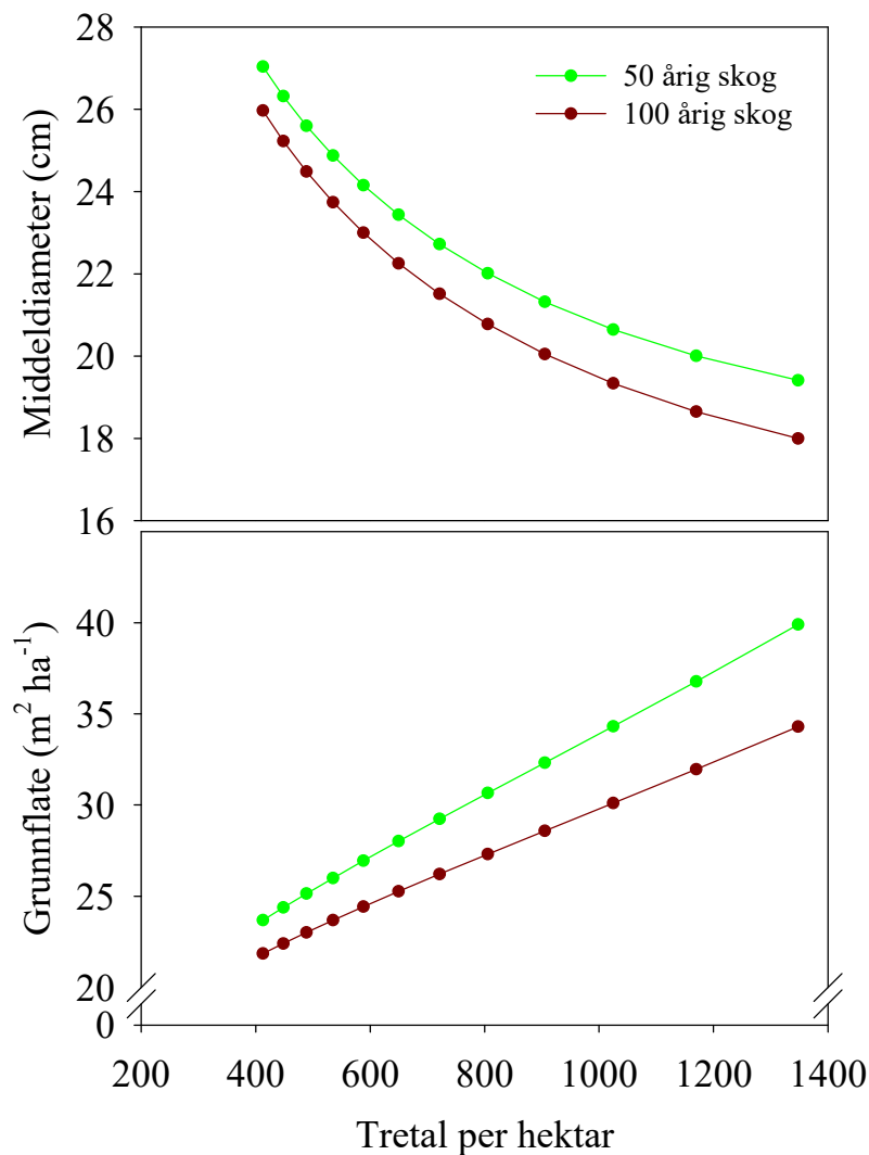
Figur 13. Predikert samband mellom tretal og middeldiameter (øvre) og tretal og grunnflatesum frå modellen for 50 og 100 år gamal skog når begge har middelhøgde 20 meter på bærlyngmark, bonitet er F17 og høgda over havet er 300 meter.
