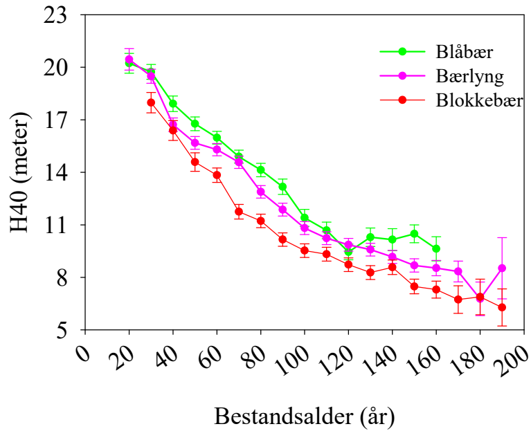
Figur 9. Bonitet i furu i høve til bestandsalder for blåbær- (øvt), bærlyng- og blokkebærskog (nedst), middel for alle høgdslag. Bonitet H40 er rekna med Tveite sin funksjon og føreset at trea har bruka normert tid for å nå brysthøgde. Pluss minus ein standardfeil er synt.
