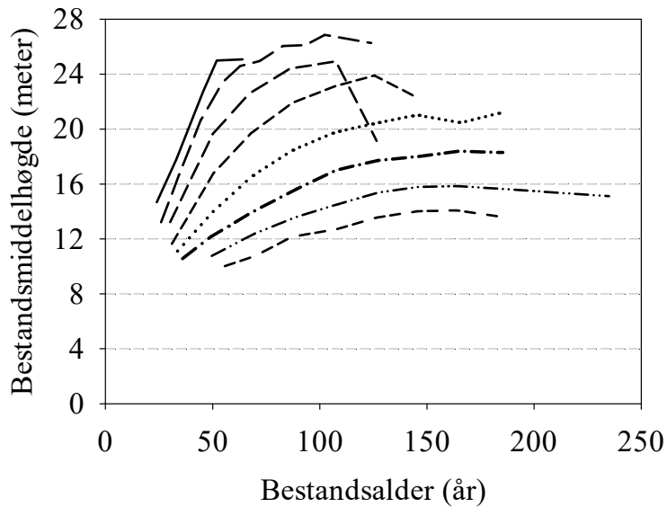
Figur 1. Arealvekta middelhøgde for gran i høve til bestandsalder i aldersklassar med 20 års breidde for bonitet G6 (nedst) til G26 (øvt).
