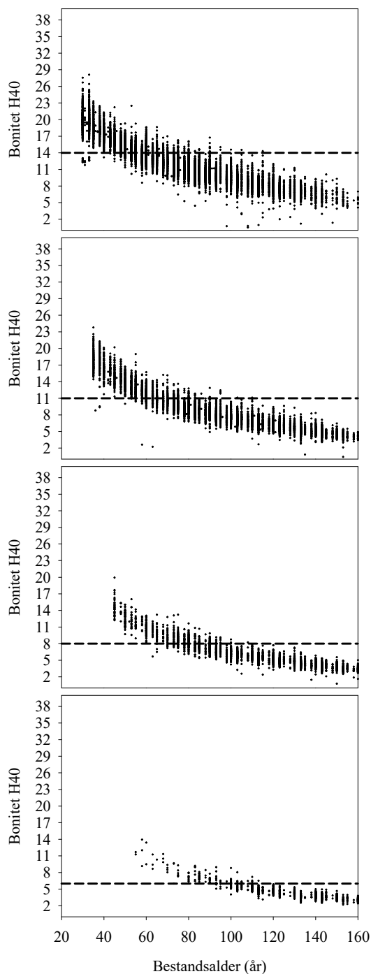
Figur 4. Bonitet H_{40_{NL}} etter (Nord Larsen m.fl. 2009) rekna på grunnlag av middelhøgde og bestandsalder for bestand klassifisert som G14 (øvtst) til G6 (nedst) i taksten. Dette er bestand der minst nitti prosent av volumet er gran.
