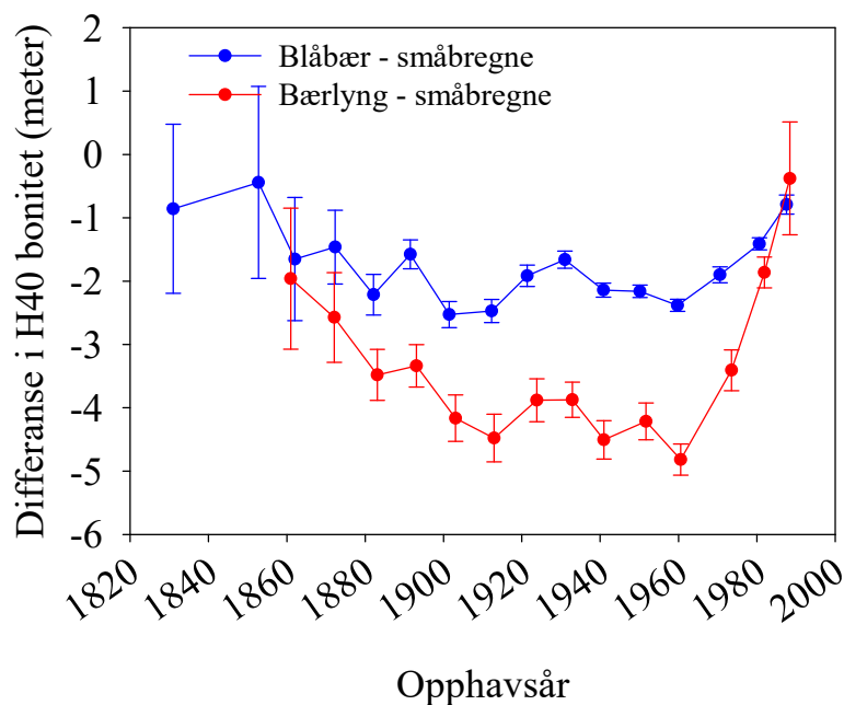
Figur 6. Differanse i H_{40NL} mellom blåbær- og småbregneskog og bærlyng og småbregneskog med opphav i ulike tiårsperiodar frå 1860. Data er frå skog frå høgdelag 400 meter over havet og bestand med minst 90 prosent gran. Tala er frå 621 bestand og 5763 dekar bærlyngskog, 6426 bestand og 64284 dekar blåbærskog, og 3626 og 40577 dekar småbregneskog. Pluss-minus ein standardfeil er synt.
