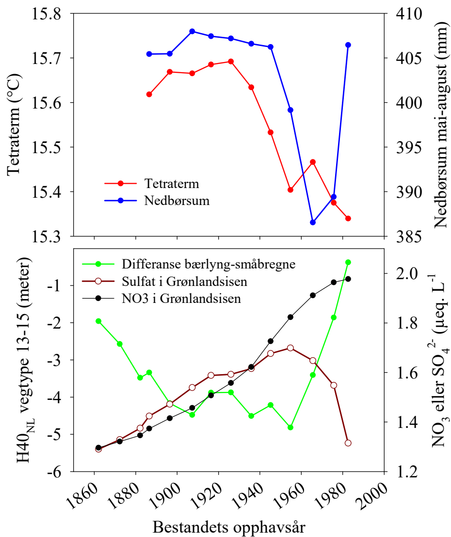
Figur 7. Øvste del gjennomsnittlige verdier for temperatur fra og med mai til og med august for perioden fra bestandets opphavsår til og med 2012, rød line, data fra e-klima for Blindern og Ås. Blå line er tilsvarende for nedbørssum med data fra Bjørnholt i Oslo fra opphavsåret til og med 2009. Nedre del er gjennomsnittlige konsentrasjoner for NO 3 og SO 4 2- i Grønlandsisen fra bestandets opphavsår til og med 2006. Data fra (Geng mfl. 2014). Grøn line i nedre figur er differansen i H40 NL bonitet mellom bærlyng og småbregneskog som også er synt i Figur 6.
