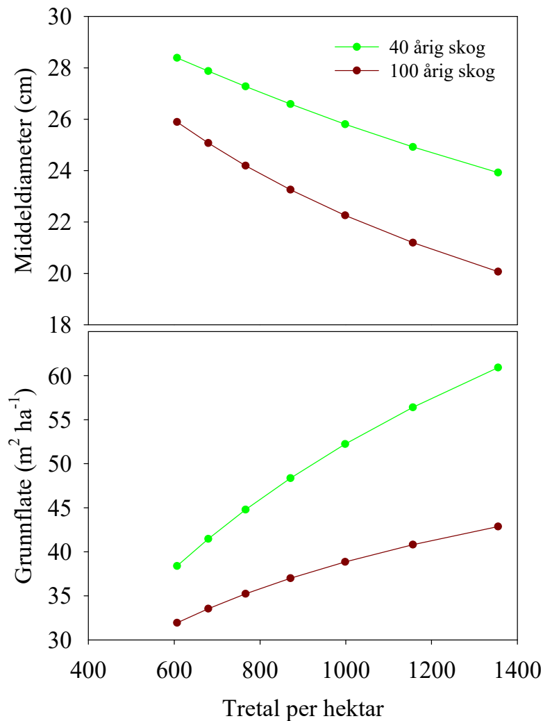
Figur 12. Predikert samband mellom tretal og middeldiameter (øvre) og tretal og grunnflatesum frå modellen for skog med opphav for 40 og 100 år sidan når begge har middelhøgde 22 meter på blåbærmark og bonitet G20.
