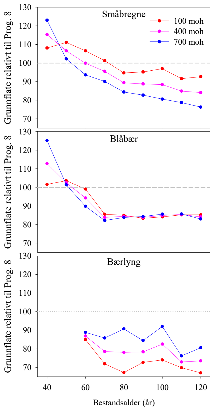
Figur 11. Estimert grunnflatesum i prosent av program 8 (sjølvtytning) i Braastad sin produksjonsmodell når bestandet har 5 prosent som føresett i program 8. Boniteten er sett til G14. Merk at raud line er 100 moh, rosa er 400 moh blå er 700 moh, medan stipla svart line markerer 100 prosent.
