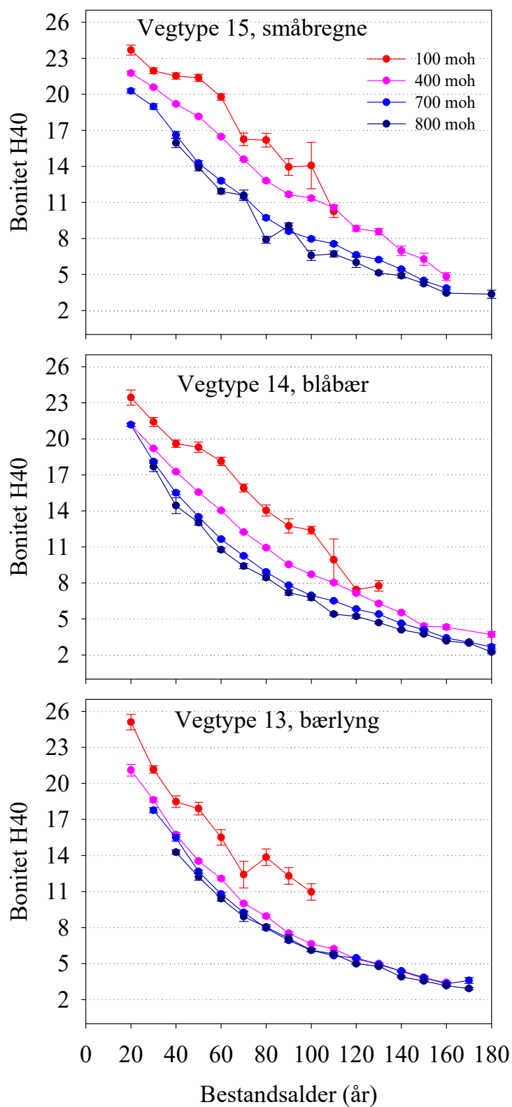
Figur 5. Arealvekta bonitet H40 NL som funksjon av bestandsalder og høgde over havet for småbregne, blåbær og bærlyngmark innan takstomårdet. Merk at høgda over havet er gjeven som nedre grense for klassen; 100-200 osv. Rosa farge indikerer 400 moh og svart 800 moh. Dette er bestand med >90% granvolum.
