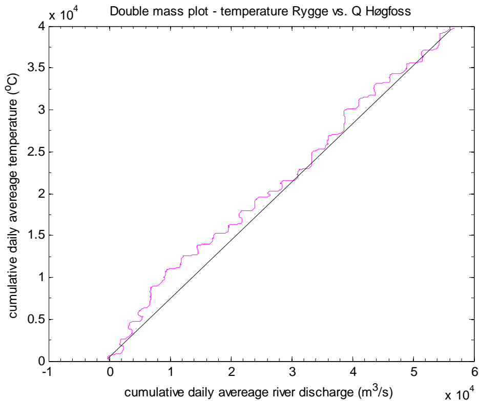
Figur 29. Akumulert døgnlige gjennomsnittsvannføring ved Høgfoss plottet mot akumulert døgnlige gjennomsnittstemperatur målt ved Rygge flyplass. Kurven viser ingen klare homogenitetsbrudd.
