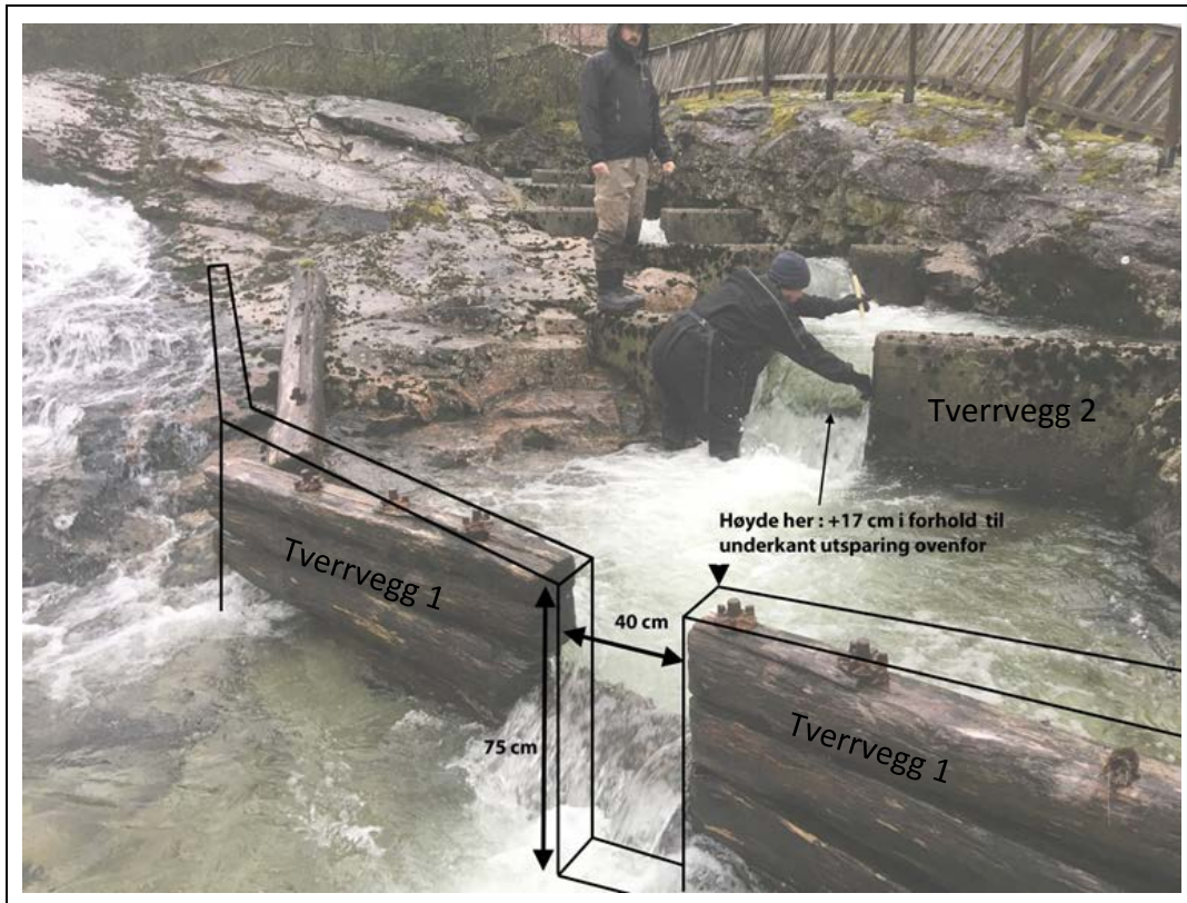
Figur 29. Prinsippkisse for utløp av trappen. Det anbefales å lage en ny tverrvegg i støpt betong som er helt tett og som har en spalteformet inngang med en bredde på 40 cm og en høyde på 75 cm. Vegghøyden økes gradvis til siden slik at det oppstår en V-formet overkant.
