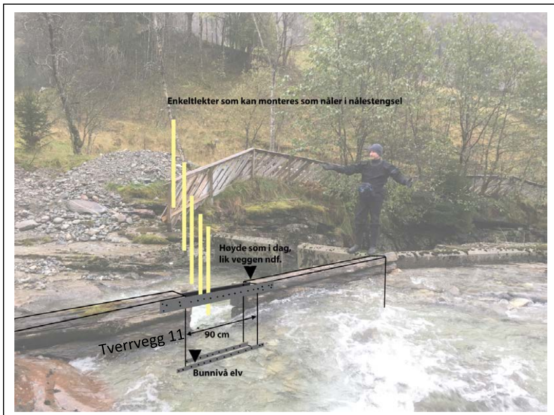
Figur 30. Prinsippkisse for vanninntaket i trappen. Det støpes en ny og tett betongvegg med spalteformet og regulerbart nålestengsel.
