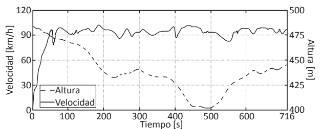
Figura 6 - CBA 5 Altura y velocidad en función del tiempo
