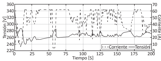
Figura 8 - Tensión y corriente en el FC stack - Ciclo CBA 5 (Zoom 200s)
