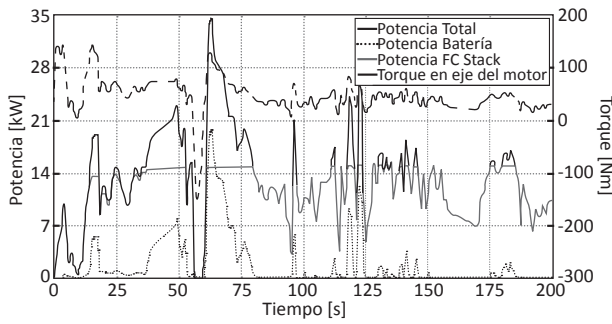
Figura 7 - Potencias y torques requeridos-Ciclo CBA 5 (Zoom 200s)
