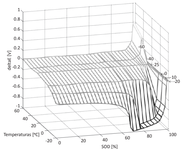
Figura 2 - a - Característica de descarga a 25°C b- delta E en función de la Temperatura y el SOD a 1°C
