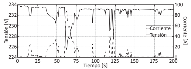
Figura 9 - Tensión y corriente en la batería - Ciclo CBA 5 (Zoom 200s)
