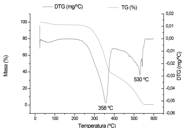
Figura 2. Curvas TGA-DTG de cáscara de maní ( Arachis hypogaea ).
