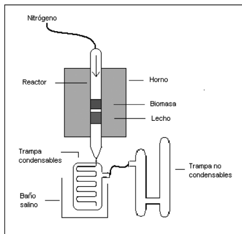
Figura 1. Esquema del sistema de reacción.
