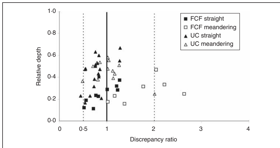
Fig. 9. Sediment discharges prediction with the Yang formula
