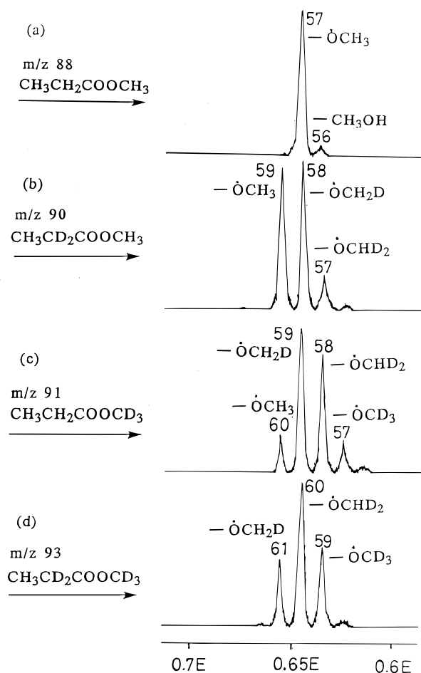
Figure 3. MIKE spectra of the molecular ions of (a) 1- d 0 ( m/z 88), (b) 1- d 2 ( m/z 90), (c) 1- d 3 ( m/z 91) and (d) 1- d 5 ( m/z 93).
