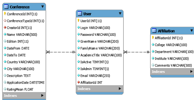
Rys. 2. Fragment diagramu ERD
