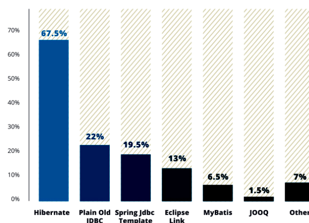
Rys. 1. Wykorzystanie technologii dostępu do danych w aplikacjach jawy [6]
