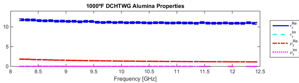
(d) Alumina 1000°F analysis using DCHTGW
