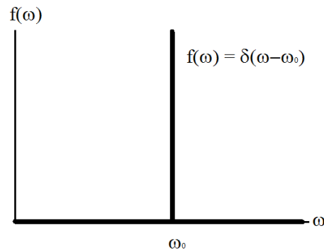
Fig. 2.1a: Dirac delta function
