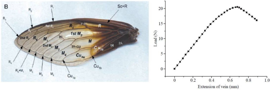
Figure 4: Cicada Vein Tensile Test [84]
