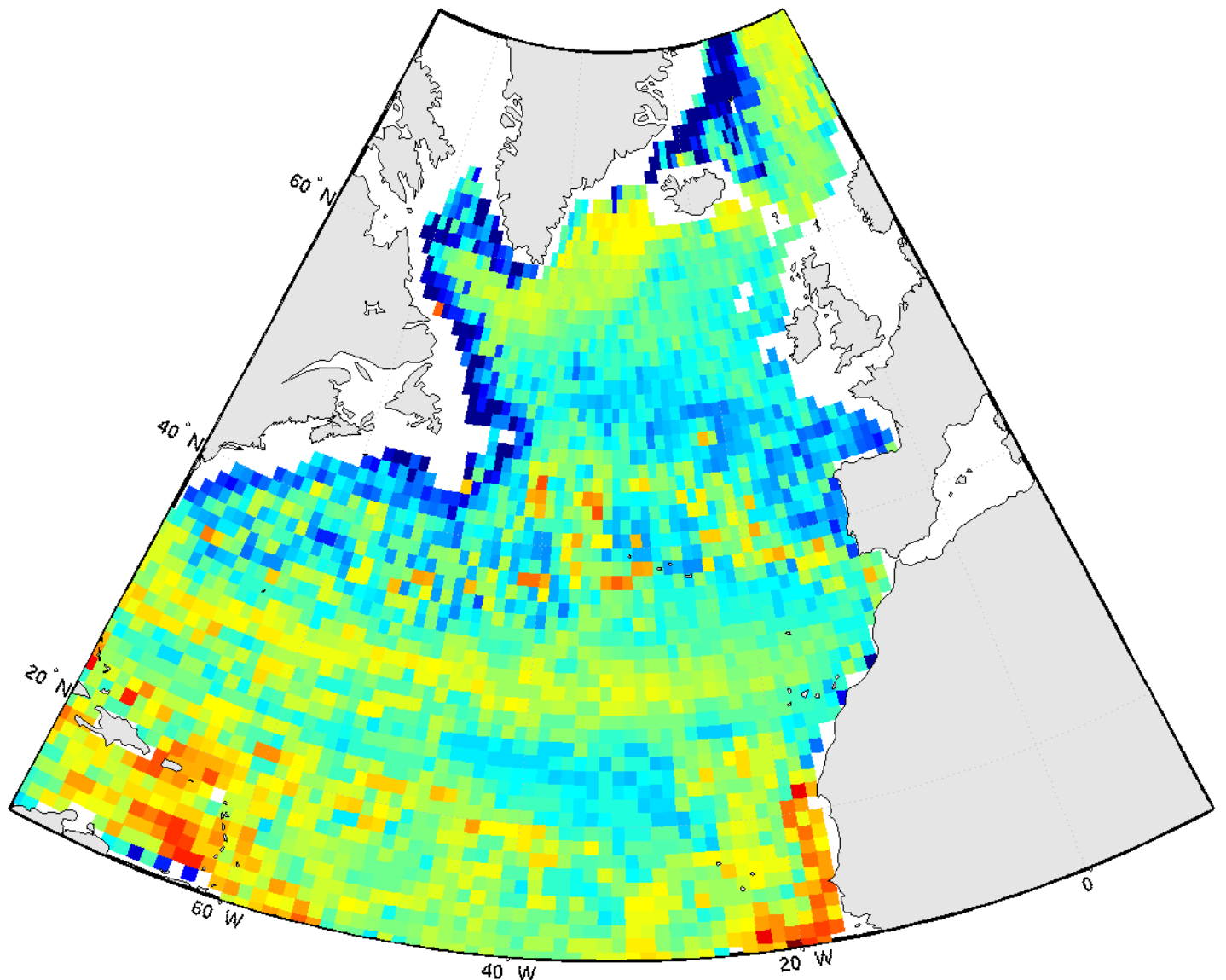
pCO 2 - april2005
