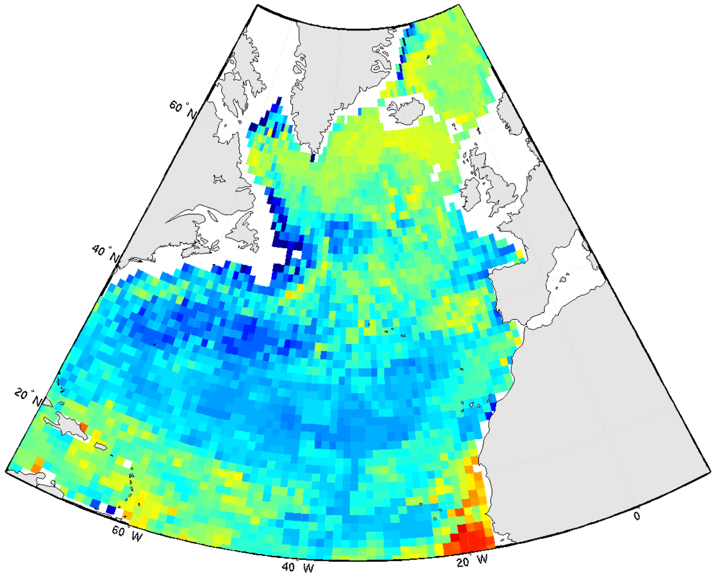
pCO 2 - april2006
