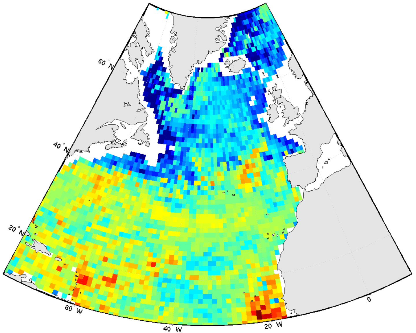
pCO 2 - may2004
