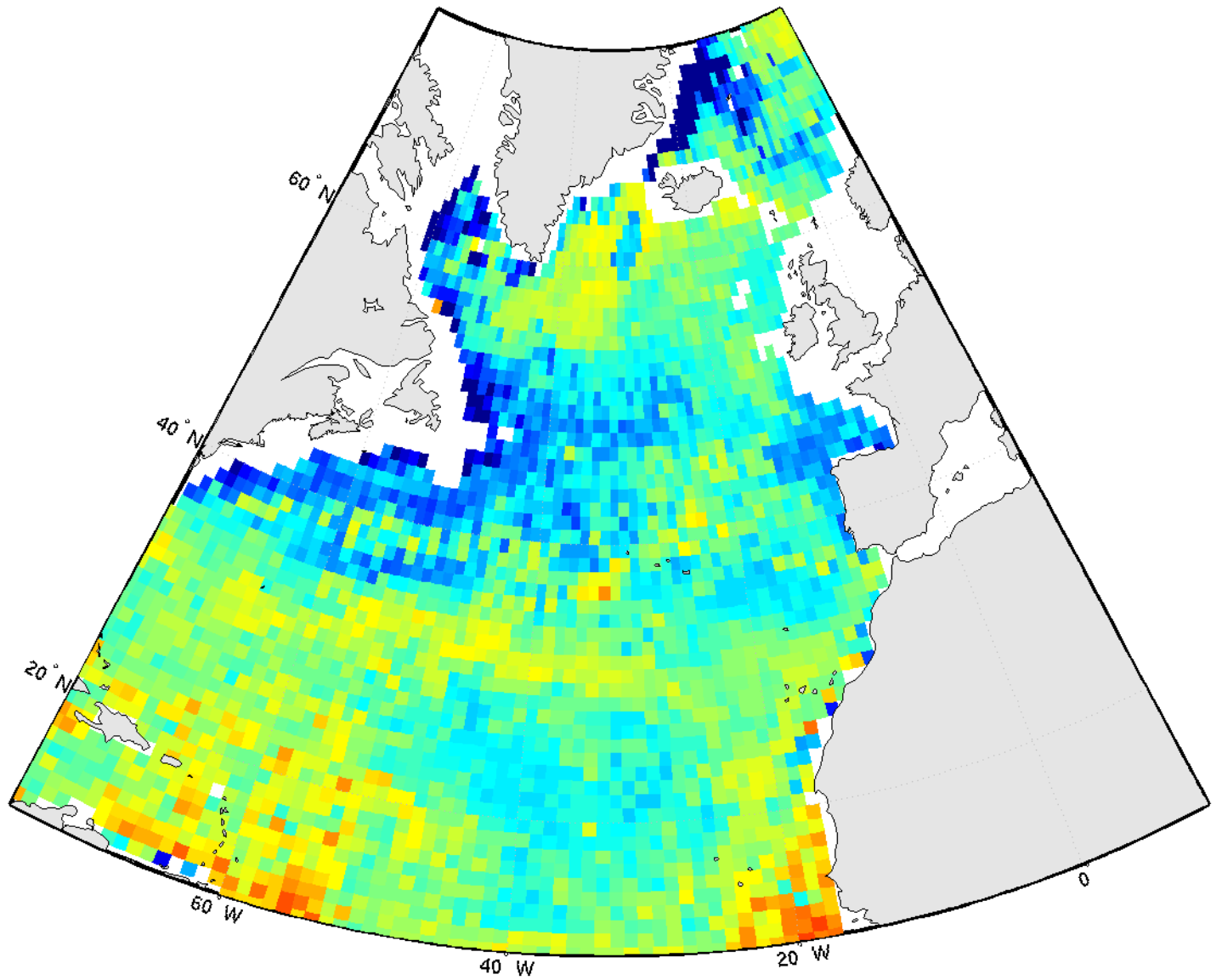
pCO 2 - april2004
