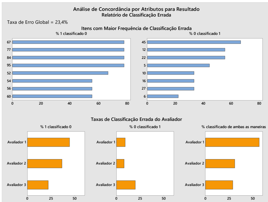
Figura 6: Relatório detalhado de Classificação a partir das respostas dos Inspetores.
