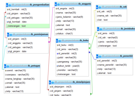
Gambar 2. Relasi antar tabel dalam database
