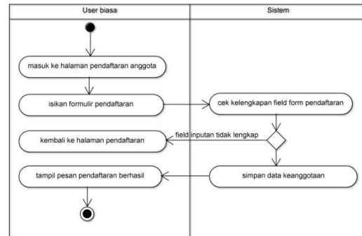
Gambar 4. Activity diagram pendaftaran anggota baru
