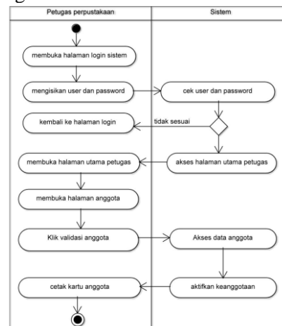
Gambar 5. Activity diagram validasi anggota
