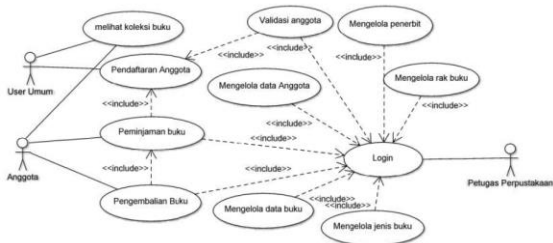
Gambar 3. Use case diagram sistem informasi yang dibangun
