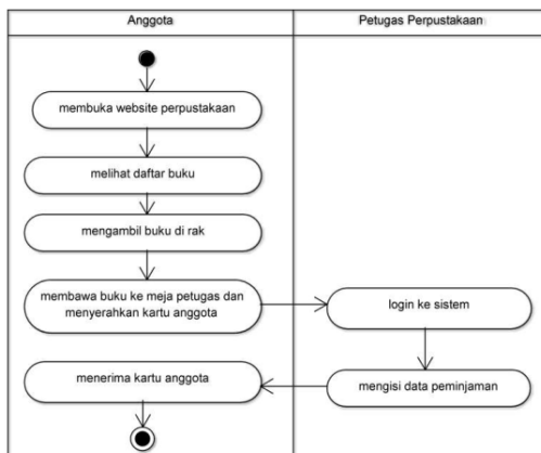
Gambar 6. Activity diagram peminjaman buku
