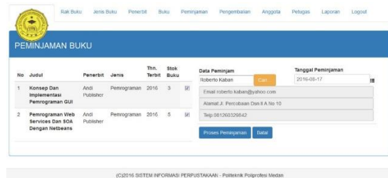
Gambar 13. Halaman peminjaman buku pada menu petugas perpustakaan
