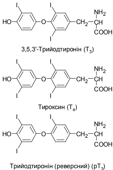
Рис. Структурні формули йодтиронінів.
