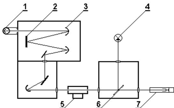
Рис. 12. Блок-схема спектрофотометра.
