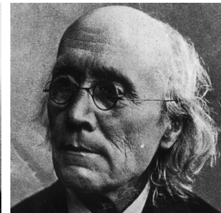
Рис. 7. Густав Фехнер.
