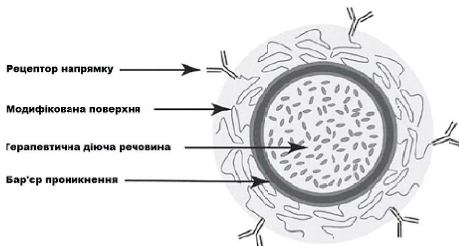
Рис. 1. Схема наночастинок, всередині якої міститься діюча речовина лікарського препарату.
