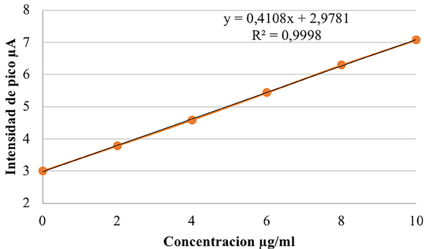
Figura 4. curva de calibración para la determinación de DCF con concentraciones (2, 4, 6, 8, 10 µg/l).
