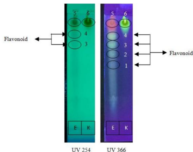
Gambar 2. Hasil KLT ekstrak etanol daun binahong ( Anredera cordifolia ) dengan fase gerak n-butanol : asam asetat : air (4:1:5) dan penampak noda AlCl 3 .
