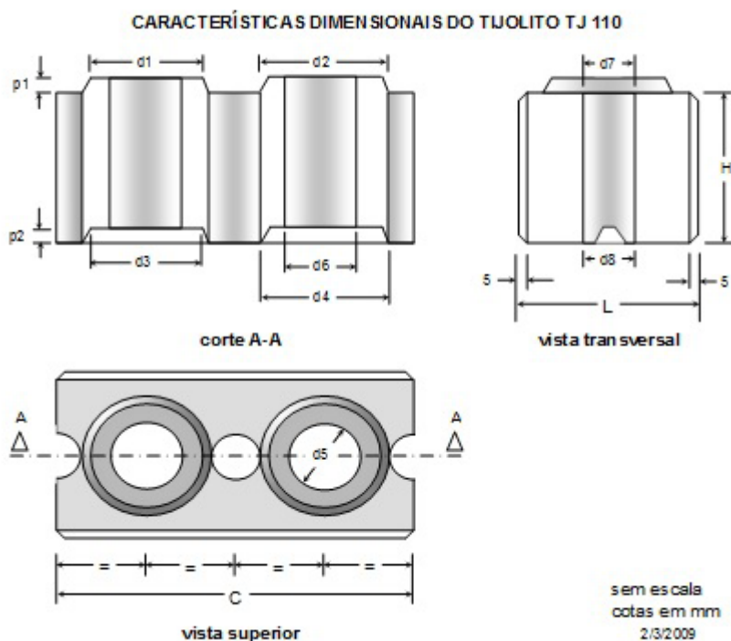
FIGURA 6 – Características dimensionais do bloco padrão. Fonte: ASSIS (2001)
