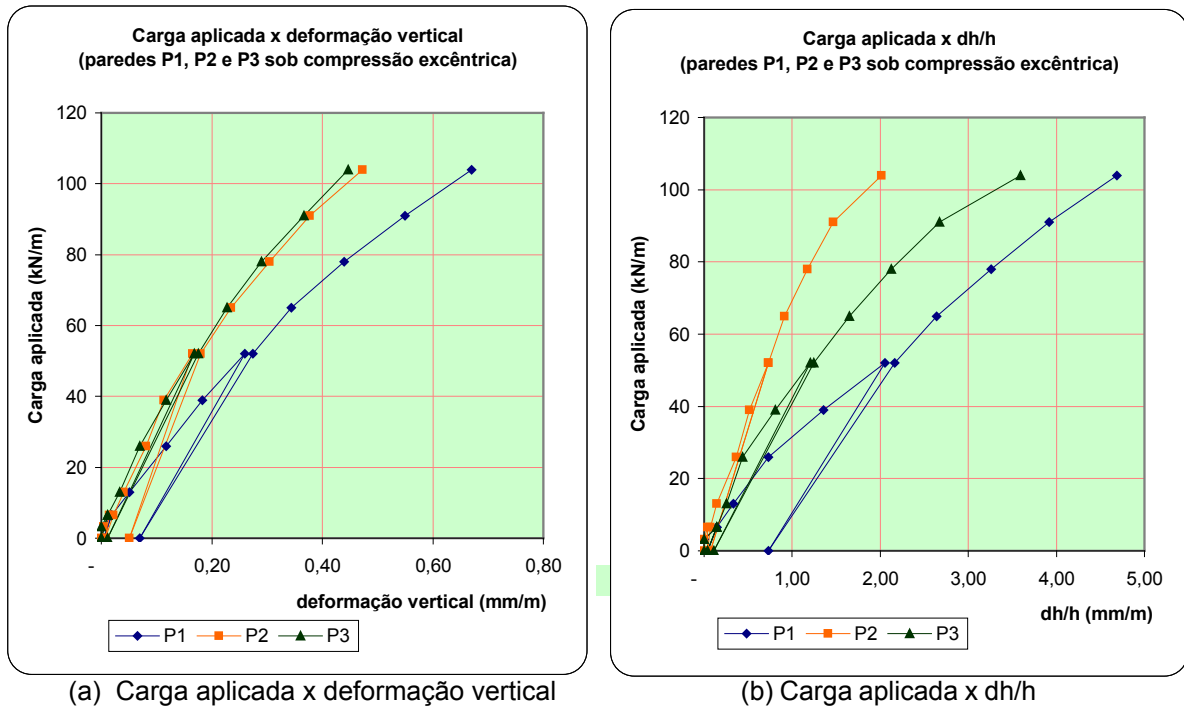
FIGURA 8 – Diagramas Carga x deformação e Carga x dh/h
