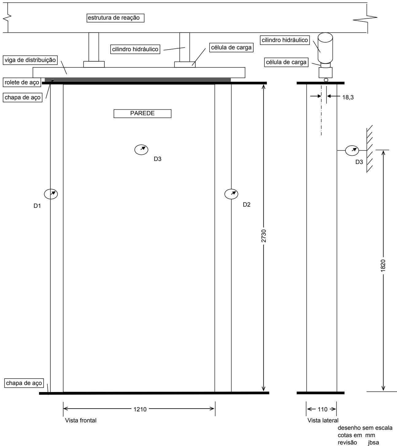
FIGURA 5 – Esquema de montagem dos instrumentos das paredes
