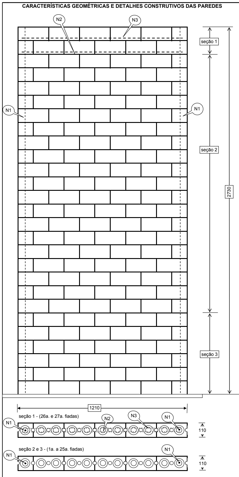
FIGURA 4 – Esquema de montagem das paredes ensaiadas à compressão excêntrica
