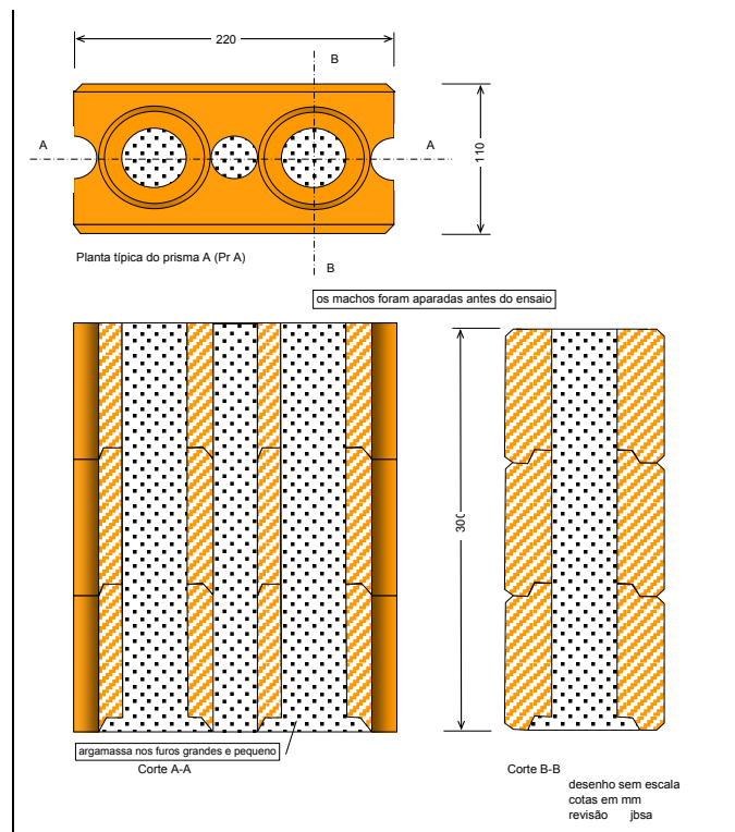
FIGURA 2 – Planta e cortes do prisma Pr A
