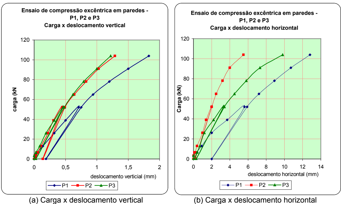
FIGURA 7 – Diagramas carga x deslocamento das paredes P1, P2 e P3
