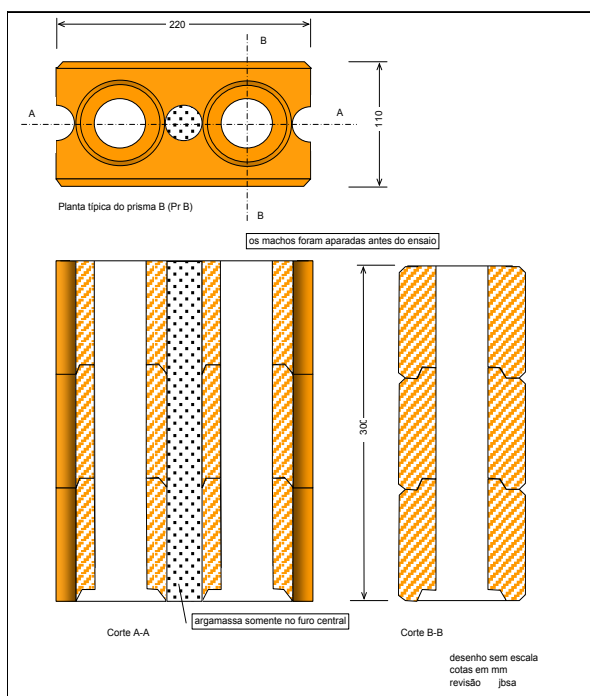
FIGURA 1 – Planta e cortes do prisma Pr B
