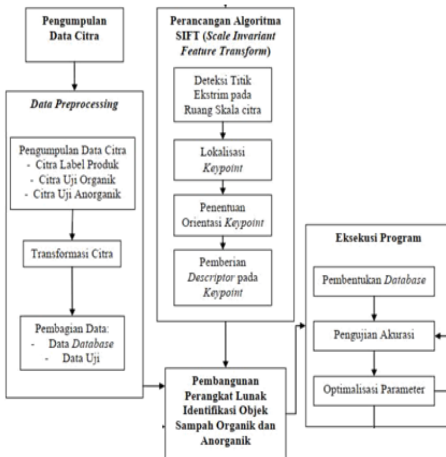
Gambar 2 : Konsep SIFT
