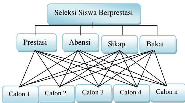
Gambar 1. Struktur Hirarki AHP
