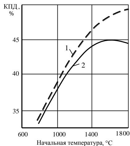
Рис. 1. Влияние охлаждения лопаток на КПД ГТУ: 1 – КПД без на охлаждения лопаток; 2 – КПД с учетом потерь энергии на охлаждение лопаток
