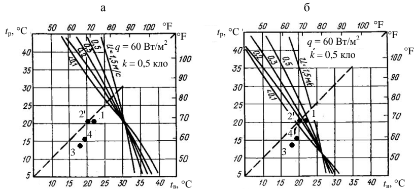
Рис. 5. Диаграммы комфорта Фангера: t_p – радиационная температура; t_b – температура воздуха; q – теплопродукция тела; u – скорость воздуха; а – q = 60 ; б – 120 \text{ Вт/м}^2
