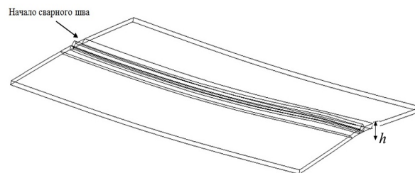
Рис. 2. Схема измерения прогиба пластины
