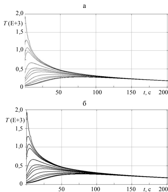
Рис. 7. Распределение температуры в средней части пластины в зависимости от времени: а – верхняя; б – нижняя поверхности; min = 30,7 °С; max = 1930,1 °С
