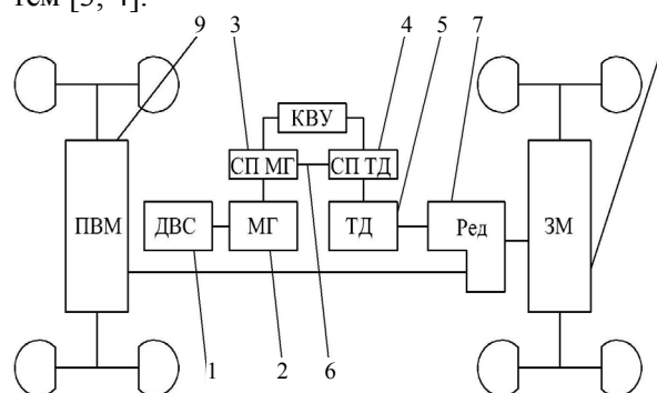
Рис. 4. Структурная схема трактора с последовательным расположением электромашин: ПВМ – передний ведущий мост; ДВС – двигатель внутреннего сгорания; МГ – мотор-генератор; ТД – тяговый электродвигатель; Ред – согласующий редуктор; ЗМ – задний мост; СП МГ – силовой преобразователь мотора-генератора; СП ТД – силовой преобразователь тягового электродвигателя; КВУ – контроллер верхнего уровня
