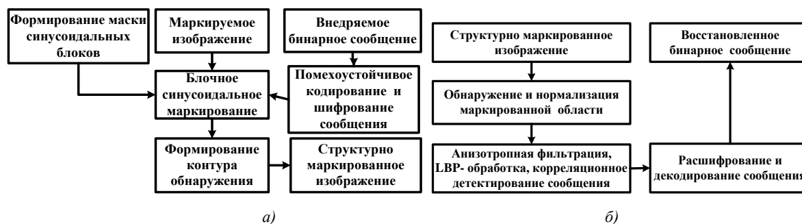
Рис. 1. Блок-схема метода блочно-структурного маркирования и считывания маркированных изображений с помощью мобильных устройств: а) синусоидальное маркирование изображений; б) текстурно-корреляционное извлечение идентификационной информации
