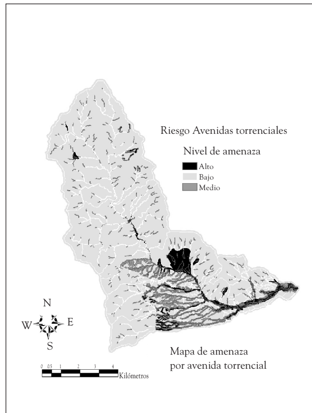
Figura 7. Asignación final de las zonas de amenaza por avenidas torrenciales, en la microcuenca de la quebrada Doña María.
