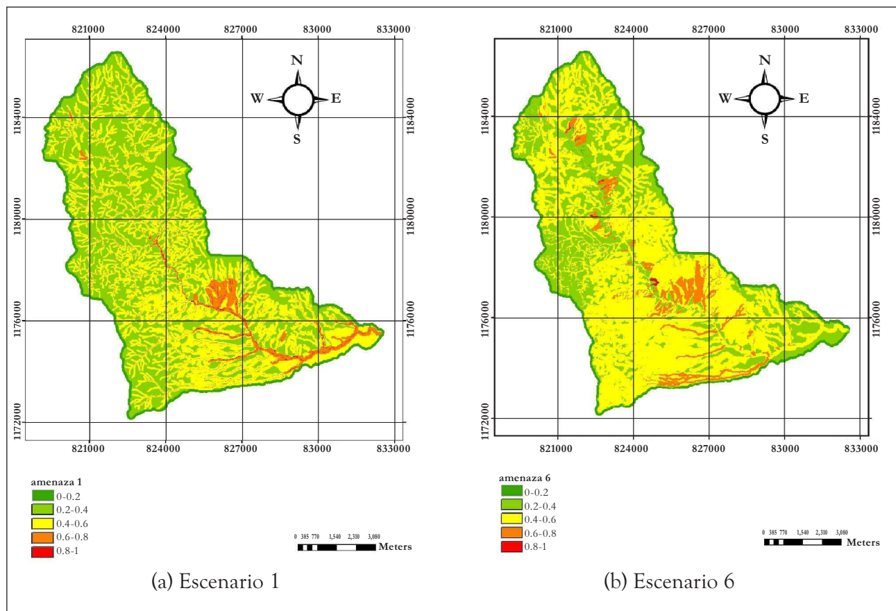
Figura 3. Mapas de amenaza con los escenarios de ponderación 1 y 6
