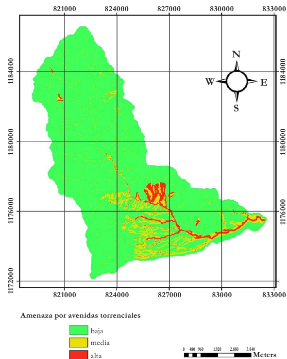
Figura 5. Mapa de amenaza por avenidas torrenciales, metodología de análisis multicriterio
