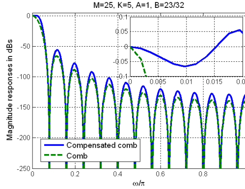
b. M=25, K=5, A=1, B=23/32
