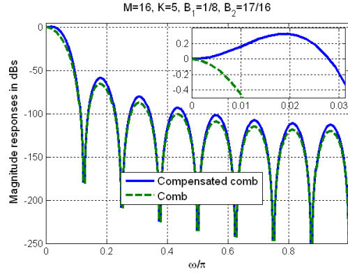
a. M=16 , K=5
