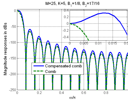
b. M=25 , K=5
