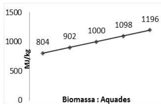
Gambar 3. Pengaruh rasio biomassa, aquades tanpa aditif terhadap slurry fuel
