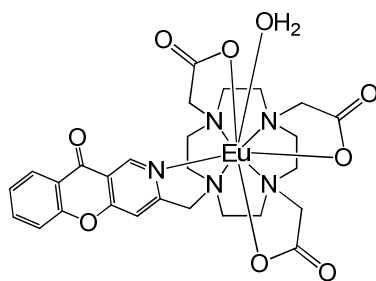
[Eu·L 1 ]
