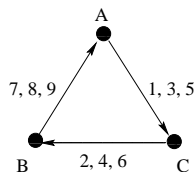
del Pezzo 0
