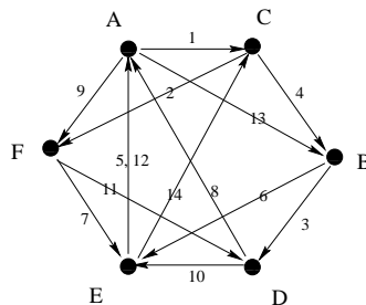
del Pezzo 3
