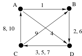
del Pezzo 1
