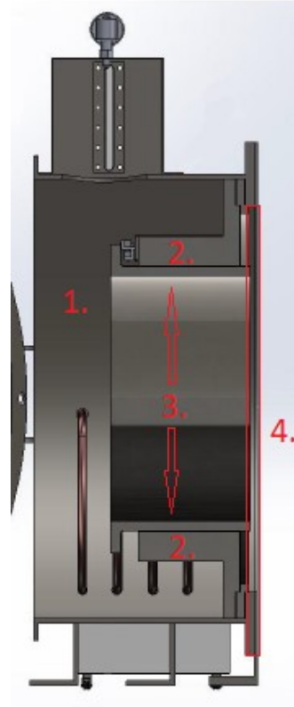
Kuva 8. Poikkileikkaus testin tärkeimmistä komponenteista (ABB 2018)
