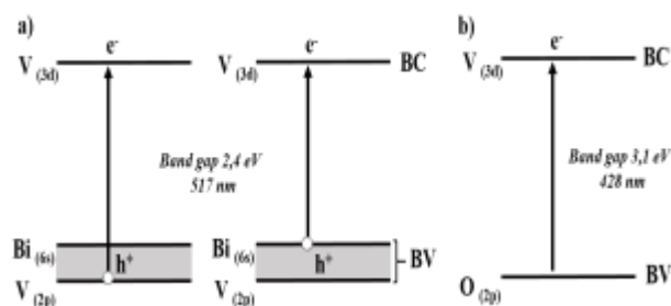
Figura 2. Diagrama de bandas do \text{BiVO}_4 nas fases (a) monoclinica scheelita e (b) tetragonal zircônia.
