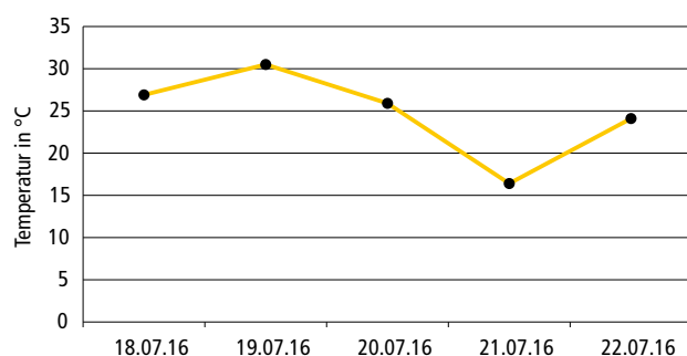
Abb. 14 | Mittlere Tagestemperaturen während des Gotthardttracks.
