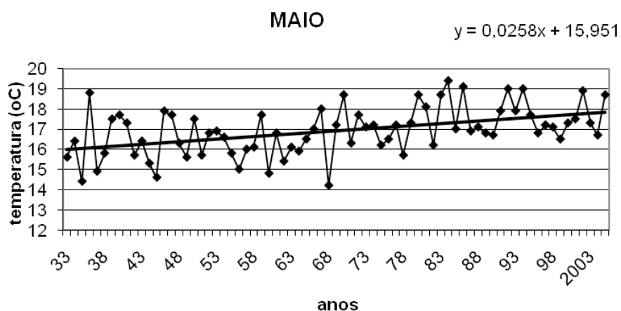
Figuras 2 e 3. Temperaturas médias dos meses de abril e maio, ao longo da série temporal do IAG-Água Funda, de 1933 até 2005, com a respectiva reta de regressão
