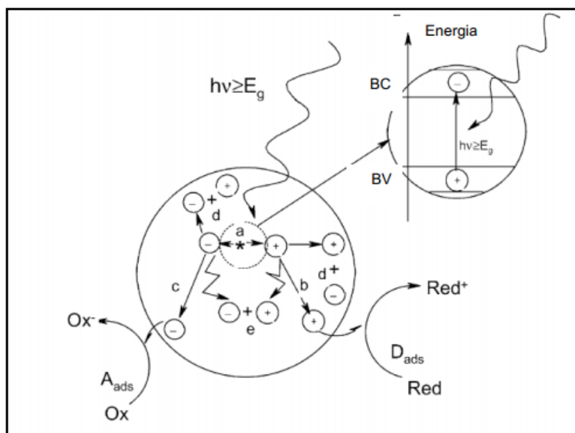
Figura 1. Principais processos ocorridos na partícula do semicondutor quando fotoexcitado: a) geração do par e_{\text{BC}}^-/h_{\text{BV}}^+ ; b) oxidação do doador (D); c) redução do aceptor (A); d) recombinação do par e_{\text{BC}}^-/h_{\text{BV}}^+ fotogerados na superfície e no cerne da partícula, respectivamente.
