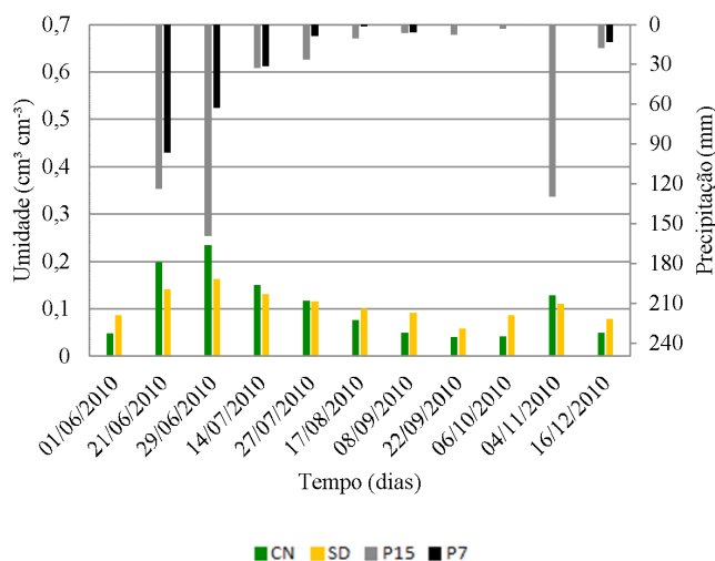
Figura 3. Distribuição temporal do conteúdo médio da água no solo Argissolo Amarelo Eutrófico abrupto para a condição de Cobertura Natural (CN) e Solo Descoberto (SD) e precipitação antecedente (ocorrida 15 (P15) e 7 (P7) dias antes do monitoramento de umidade) para o período de junho a dezembro de 2010
