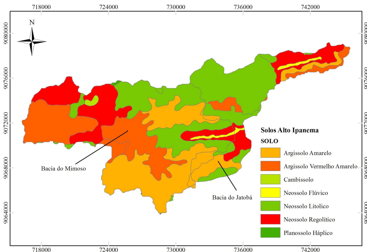
Figura 1. Mapa de solos da Bacia Representativa do Alto Ipanema com delimitação das Bacias Experimentais do Jatobá e Mimoso e os tipos de solo presentes
