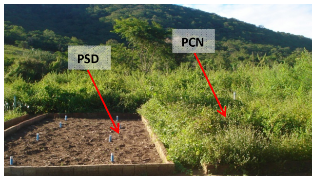
Figura 2. Parcelas experimentais com Solo Descoberto (PSD) e Cobertura Natural (PCN)
