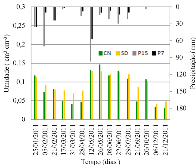
Figura 4. Distribuição temporal do conteúdo médio da água no solo Argissolo Amarelo Eutrófico abrupto, sob condições de Cobertura Natural (CN) e Solo Descoberto (SD) e precipitação antecedente (ocorrida 15 (P15) e 7 (P7) dias antes do monitoramento de umidade) para os meses do ano de 2011
