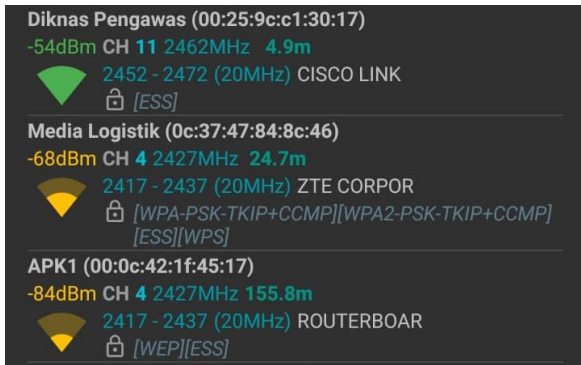
Gambar 12. Pengukuran pada Ruang Pengawas pada Jarak 5 Meter
