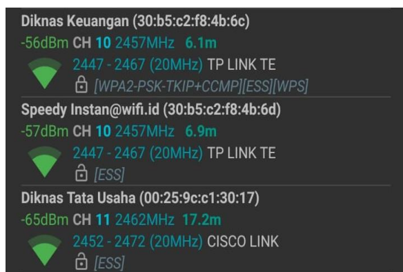
Gambar 6. Pengukuran pada Ruang Diknas Keuangan
