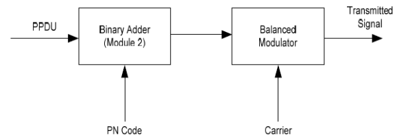
Gambar 1. Blok Modulasi DSSS [6]
