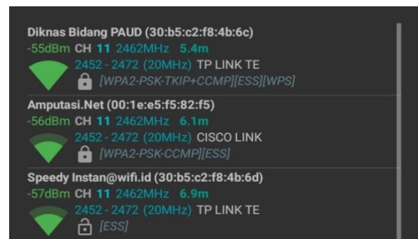
Gambar 10. Pengukuran pada Ruang Bidang PAUD Jarak 5 Meter
