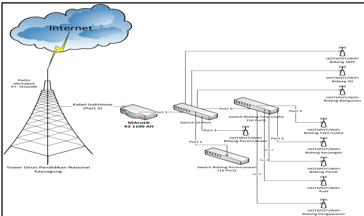
Gambar 4. Topologi WLAN Diknas Kayuagung
