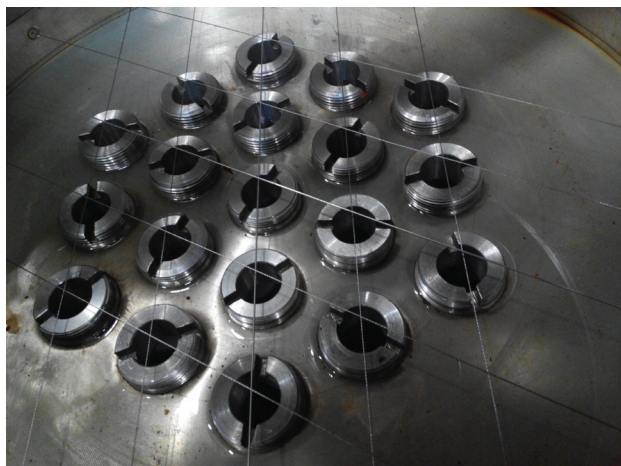
Рисунок 4 – Сетчатый и стержневой типы пространственных кондуктометрических датчиков
