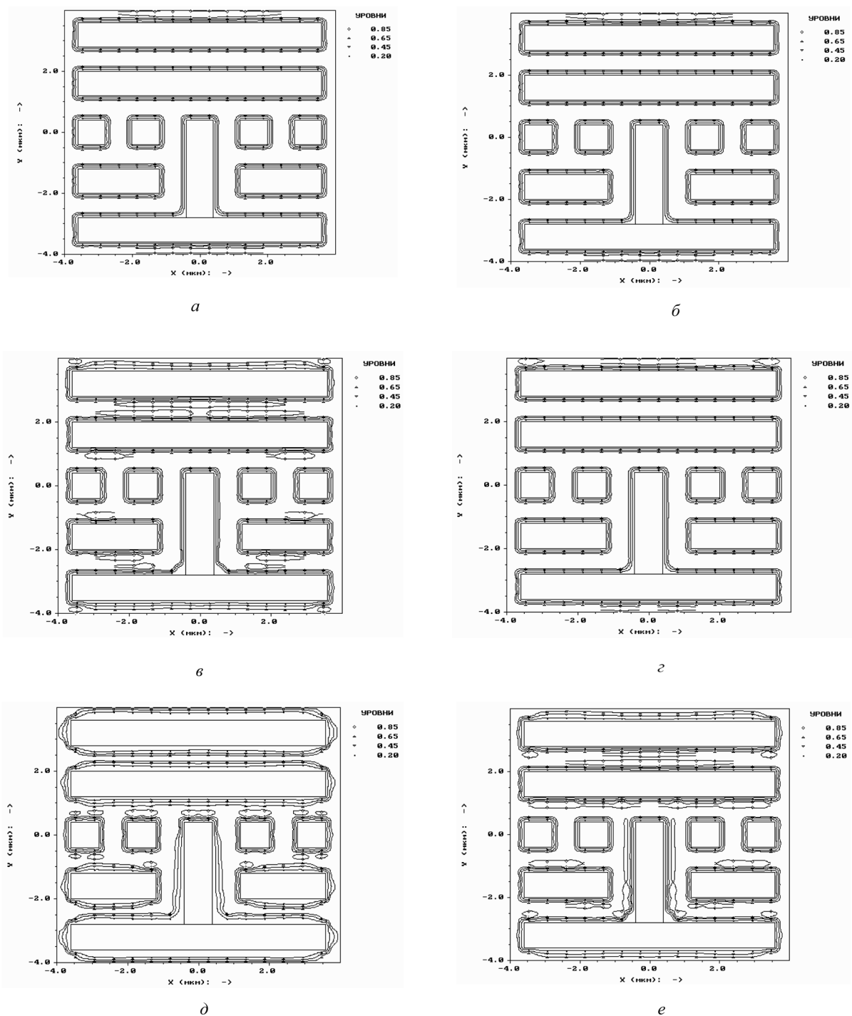
Рис. 2. Зависимость качества формирования элементов с номинальной шириной 0,8 мкм при разных степенях расфокусировки объектива \Delta f (мкм): 0 (а); \pm 0,25 (б); +0,5 (в); -0,5 (г); +1,0 (д); -1,0 (е)
