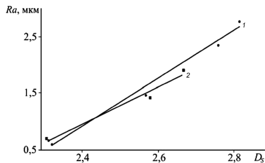
Рис. 6. Зависимость шероховатости обработанной поверхности Ra напыленных покрытий от величины фрактальной размерности совокупности механических свойств D_s : 1 – газопламенное, из порошковой проволоки Fe_{80}B_{20} ( D_s = 2,32 ); электродуговое, из порошковых проволок Fe_{80}B_{20} ( D_s = 2,57 ), Fe_{79}Cr_{16}B_5 ( D_s = 2,68 ); газопламенное, порошками Fe_{80}B_{20} ( D_s = 2,76 ), Fe_{79}Cr_{16}B_5 ( D_s = 2,82 ); 2 – газопламенное, порошком Fe_{78}B_{10}Si_{12}
