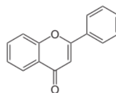
Gambar 2. Struktur flavan.
