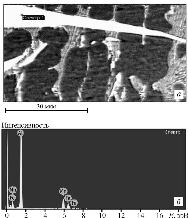
Рис. 6. Первичные кристаллы фазы Al_6(Fe, Mn) в сплаве 4 (см. табл. 1)
