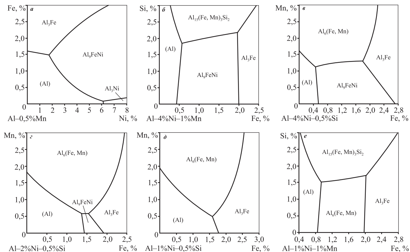
Рис. 1. Проекция поверхности ликвидуса в сечениях системы Al–Ni–Mn–Fe–Si
