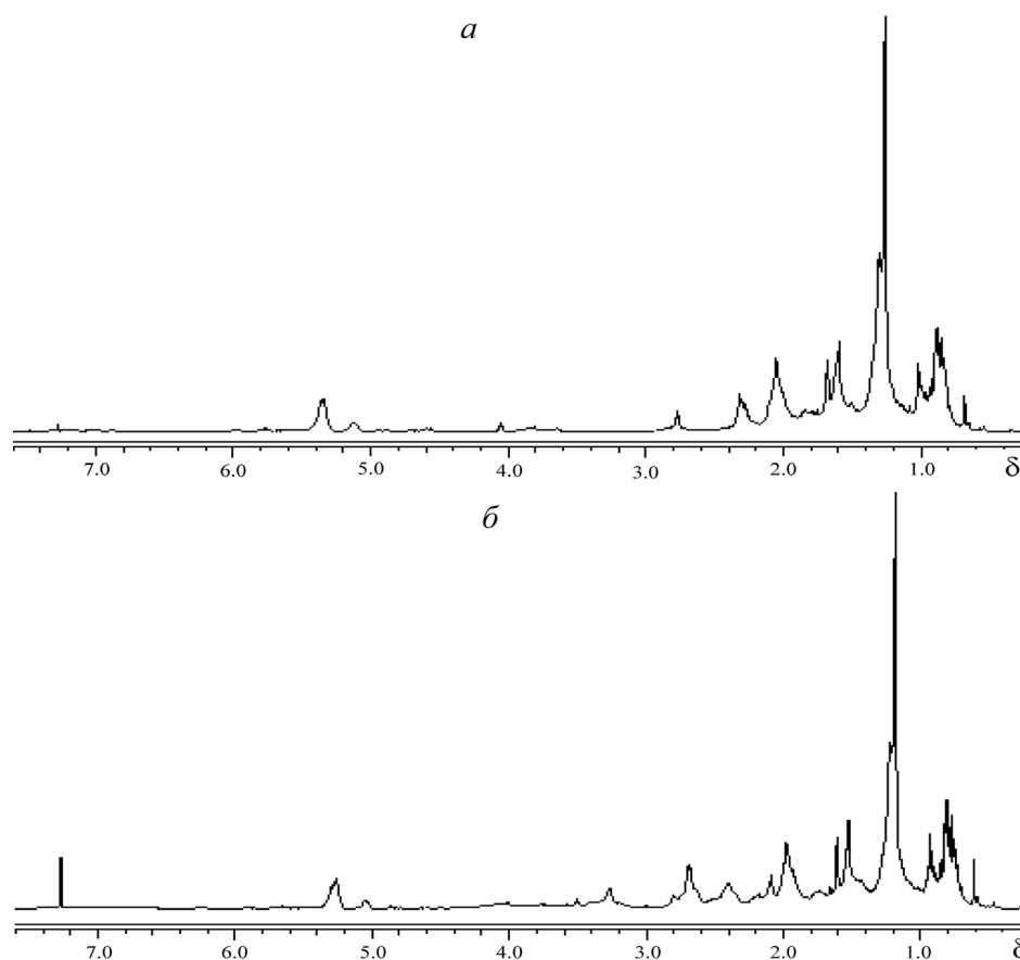
1 Н ЯМР спектры таллового пека: а – чистый талловый пек, б – талловый пек, модифицированный 30 мас.% полиэтиленполиамином
