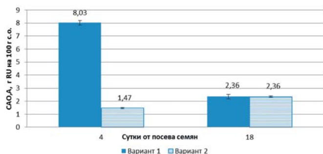
Рис. 5. Антиоксидантная активность микрозелени брокколи при проращивании на свету и в темноте Fig. 5. Antioxidant activity of broccoli microgreen when germinating in the light and in the dark
